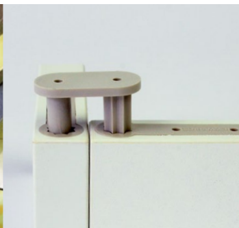
Einstecken des U-Verbinders Inserting of the U- push-fit connector
